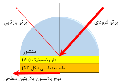
شکل ۱: کریستال مگنتوآپتیکی بر پایه پیکربندی کرچمن.
