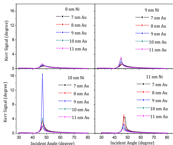
شکل ۳: سیگنال کر در پیکربندی کرچمن برای ساختار شیشه/طلای نیکل در ضخامت‌های مختلف طلا و نیکل به ازای زاویه‌های ۳۰ تا ۹۰ درجه تابش فرودی رسم شده است.
