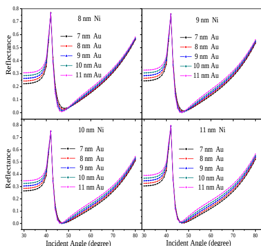
شکل ۲: بازتاب از ساختار شیشه/طلای نیکل در پیکربندی کرچمن در ضخامت‌های مختلف طلا و نیکل به ازای زاویه‌های ۳۰ تا ۹۰ درجه تابش فرودی.
