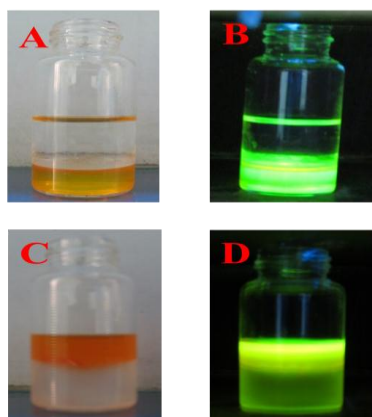
شکل ۲: تصاویر مربوط به روند انتقال فاز نانوذرات کادمیم تلوراید از آب به دودکانتیول تحت نور محیط (A و C) و تابش نور لامپ ماوری بنفش (B و D): A و B تصاویر مربوط به نانوذرات در آب با گسیل نورتابی سبز همراه با دودکانتیول و استن. C و D تصاویر مربوط به نتایج بعد از تعویض لیگاند و انتقال نانوذرات از آب به دودکانتیول
