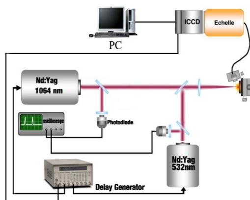
شکل ۱: چیدمان آزمایش
