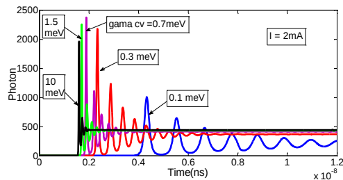
شکل ۷: تحولات زمانی فوتونها در جریان تزریقی ۲ میلی آمپر و پهن شدگی همگن با ۱/۵، ۰/۷، ۰/۳، ۰/۱، FWHM و ۱۰ meV.
