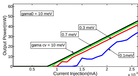
شکل ۲: نمودار توان خروجی بر حسب جریان تزریقی با در نظر گرفتن پهن شدگی ناهمگن با FWHM، ۱۰ meV و پهن شدگی همگن با FWHM، ۰/۱، ۰/۳، ۰/۷ و ۱۰ meV.
