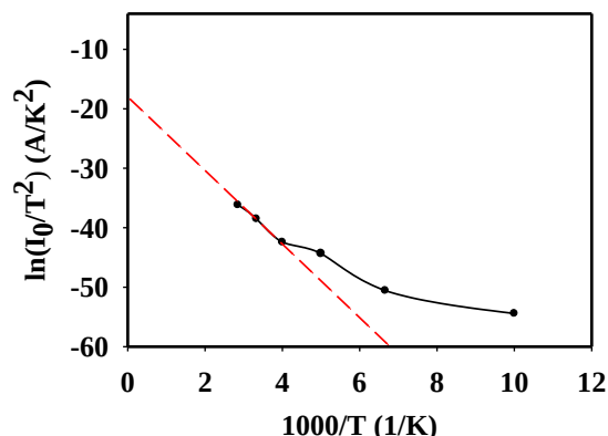
شکل ۳: نمودار ریچاردسون وابسته به تغییرات \ln(I_0/T^2) بر حسب 1000/T مربوط به دیود شاکتی Au/n-GaN
