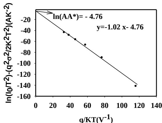
شکل ۴: نمودار اصلاح شده ریچاردسون مربوط به دیود شاکتی Au/n-GaN
