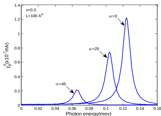
شکل ۲: تغییرات ضریب OR بر حسب انرژی فوتون فرودی، برای مقادیر مختلف پارامتر \alpha_0 .
