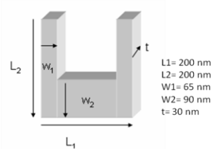
شکل ۳: چیدمان فضای محاسباتی.
