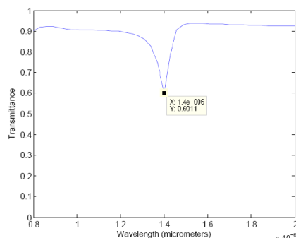
شکل ۵: نمودار انتگرال چگالی انرژی براساس طول موج برای ساختار SRR شبیه‌سازی شده.
