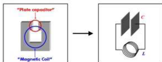
شکل ۱: تناظر مدار LC و ساختار SRR.
