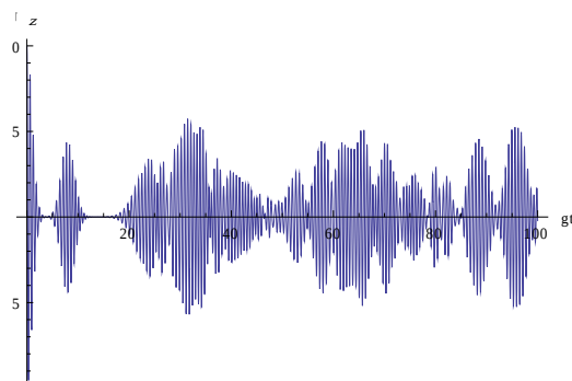
شکل ۲: تحول زمانی وارونی اتمی \langle \sigma_z \rangle برای برهم کنش اتم با میدان در حالت برهم نهی شده بر حسب زمان بهنجار شده \tau = gt و به ازای \Delta = 0 ، \varphi = \frac{\pi}{2} و |\alpha|^2 = 25
