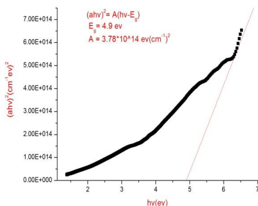
شکل ۴ تغییرات (h\nu)^2 برحسب h\nu
