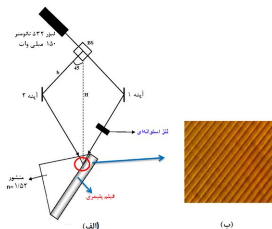
شکل ۳-الف) شمای کلی دستگاه نویسنده توری کج. عدسی استوانه-ای در مسیر پرتوی دوم باعث کاهش اندازه نقطه این پرتو می‌شود. BS: جداساز پرتو (ب) تصویری از یک توری حجمی با دوره تناوب ۱ میکرون که توسط روش هولوگرافی ایجاد شده.
