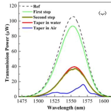
شکل ۴. (الف) طیف عبوری تیپ ساخته شده با قطر نهایی ۱ \mu\text{m} اسید در (P_i)_{\text{max}} \sim P_0/10 خارج شده است (ب) تیپ با قطر نهایی ۲ \mu\text{m} ، اسید در (P_i)_{\text{max}} \sim P_0/2.5 خارج شده است.
