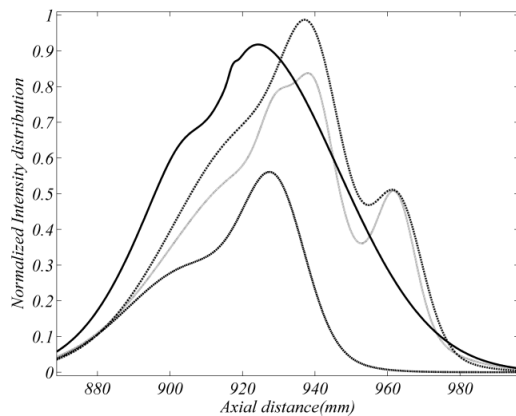
شکل ۶: توزیع شدت محوری تجربی، اکسیلن بر پایه‌ی غربال فوتونی با توزیع کلاسیک (خط ممتد)، توزیع گاوسی با N_0=650 (خط چین)، توزیع گاوسی با N_0=850 (نقطه‌چین)، توزیع گاوسی با N_0=1000 (خط نقطه).
