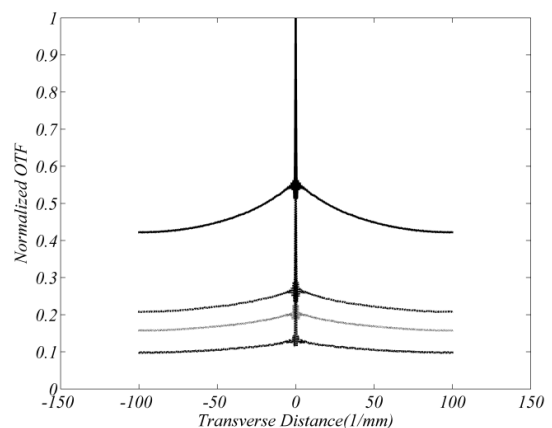
شکل ۸: محاسبه عددی تابع انتقال اپتیکی بهنجار (OTF)، اکسیلن بر پایه‌ی غربال فوتونی با توزیع کلاسیک (خط ممتد)، توزیع گاوسی با N_0=650 (خط چین)، توزیع گاوسی با N_0=850 (نقطه‌چین)، توزیع گاوسی با N_0=1000 (خط نقطه).
