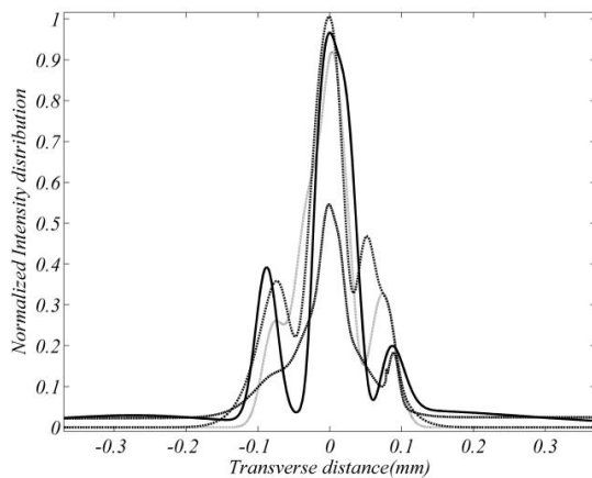
شکل ۷: توزیع شدت عرضی تجربی، اکسیلن بر پایه‌ی غربال فوتونی با توزیع کلاسیک (خط ممتد)، توزیع گاوسی با N_0=650 (خط چین)، توزیع گاوسی با N_0=850 (نقطه‌چین)، توزیع گاوسی با N_0=1000 (خط نقطه).
