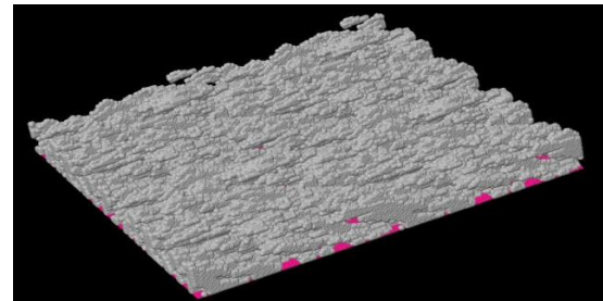
شکل ۴- نتایج شبیه سازی در زاویه \alpha = 86^\circ و \Delta\alpha = 4^\circ
