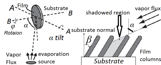
شکل ۲- دستگاه لایه نشانی بخار نشست مایل (PVD)
