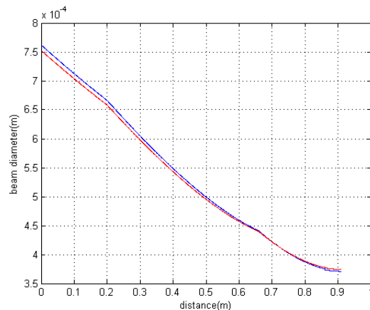
شکل ۱- نمودار تغییر قطر پرتو برای فواصل مختلف طول بازآواگر ردیف ۳ جدول ۱.
