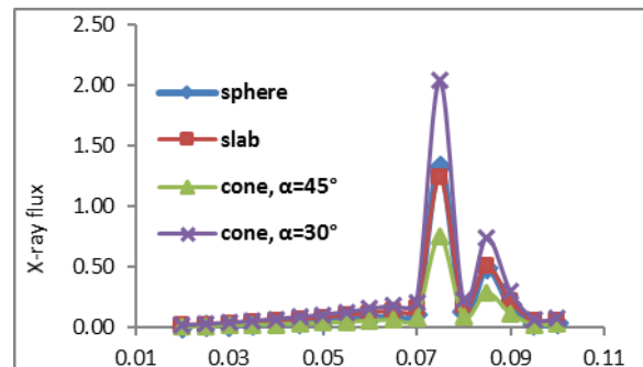
شکل ۴: مقایسه شار اشعه ایکس با سه هدف تیغه ای، مخروطی و کروی شکل سربی با t=h=d=1500\mu\text{m} ؛ دو زاویه راس مخروط \alpha=30^\circ و \alpha=45^\circ .
