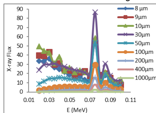
شکل ۲: شار اشعه ایکس حاصله با هدف کره سربی با قطرهای مختلف.
