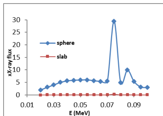
شکل ۵: مقایسه دو هدف تیغه ای و کروی در t=d=100\mu\text{m} .
