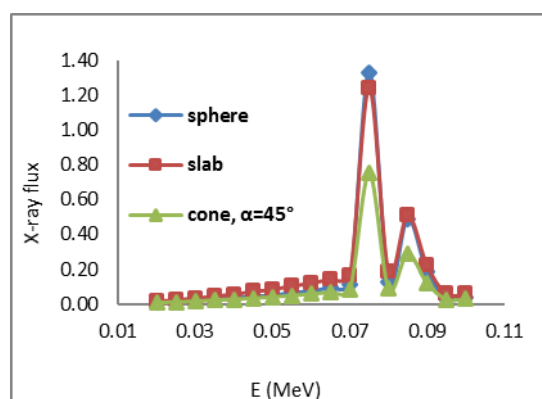
شکل ۳: مقایسه شار اشعه ایکس با سه هدف تیغه ای، مخروطی و کره ای شکل سربی با h=d=2000 \mu\text{m} ؛ بالا: \alpha=30^\circ و پایین: \alpha=45^\circ .
