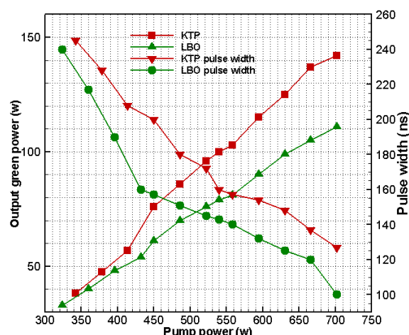
شکل ۶: توان خروجی لیزر سبز در حضور بلور KTP و LBO
