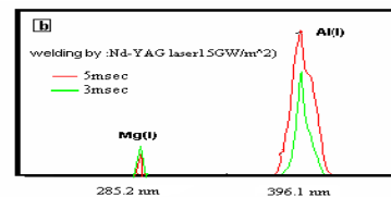
شکل ۳. دو خط مشخصه تابشی، برای دو فلز جوش در پهنای پالسی متفاوت ۳ و ۵msec و چگالی توان تابشی ۱۵GW/m²
