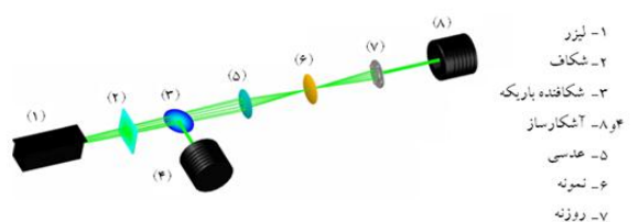
شکل ۱: چیدمان آزمایشگاهی اندازه‌گیری حدنوری.
