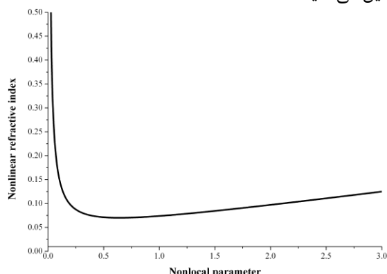
شکل ۳: وابستگی ضریب شکست غیرخطی محیط به تغییرات مقدار پارامتر غیرموضعی. مقدار \Delta T_{p-v} برابر با 0.3 فرض شده است.
