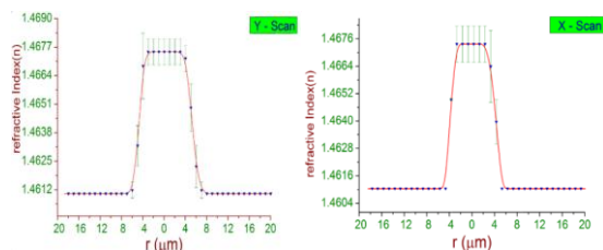
شکل ۴: جاروب سطح مقطع فیبر در جهت X و Y
