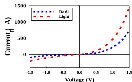
شکل ۵: مشخصه I-V وابسته به پیوندگاه p-CuO/n-ZnO در شرایط تاریکی و نورتابی.
