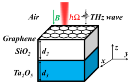
شکل ۱: شماتیکی از ساختار لایه‌ای که تحت تأثیر میدان مغناطیسی (B)، نور لیزر هلیوم-نئون ( \hbar\Omega ) و موج الکترومغناطیس (THz wave) قرار گرفته است.
