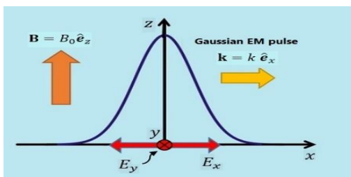
شکل ۱: پیکربندی هندسی موج X در پلاسما مغناطیبه
