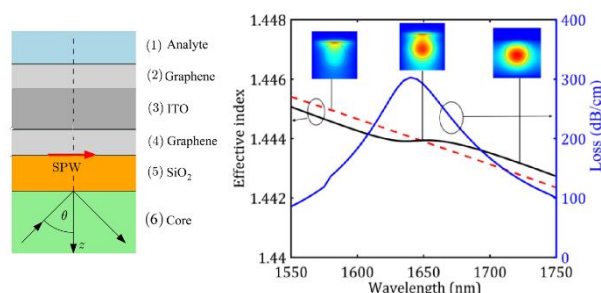
شکل ۷: شماتیک حالت سوم به همراه نمودار تلفات و ضریب شکست موثر برای مدهای مغزی و SPP به ازای ضریب شکست آنالیت 1/33 .
