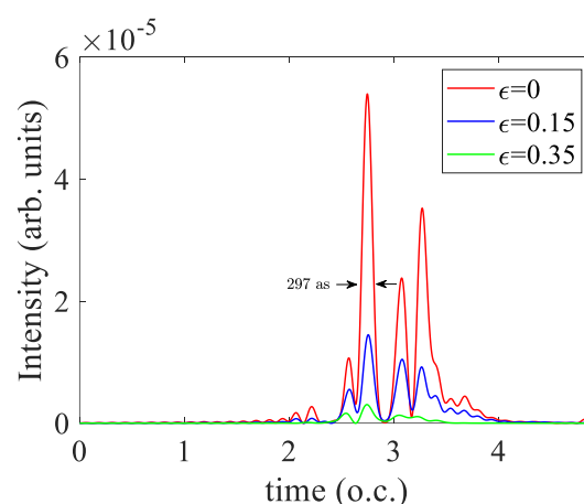
شکل ۴: تپ‌های آتوانیه حاصل از برهم‌نهی هماهنگ‌های مرتبه ۱۸ ام تا ۲۶ ام در برهم‌کنش مولکول کلرین با پالس‌های قطبیده خطی و بیضوی.
