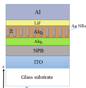
شکل ۳: ساختار OLED با نانومیل به صورت شماتیک
