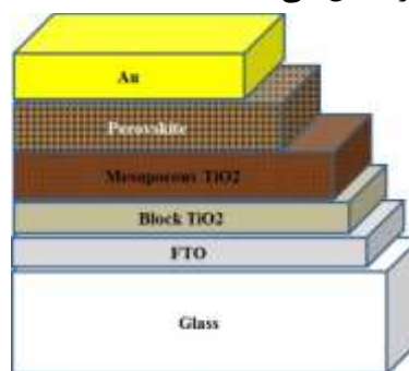
شکل 1: طرح شماتیک از سلول خورشیدی پروسکایتی
