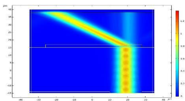
شکل ۷: جفت‌کننده ورودی عبوری بهینه شده با ضخامت ۲ میکرومتر
