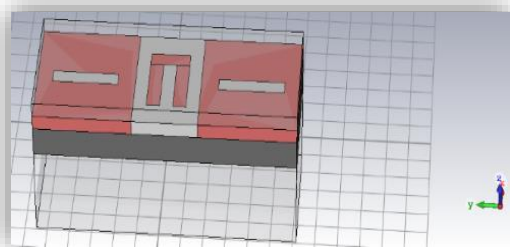
شکل ۲: طراحی ساختار حسگر به صورت عدد پی در نمونه و میله‌های افقی در صفحات.
