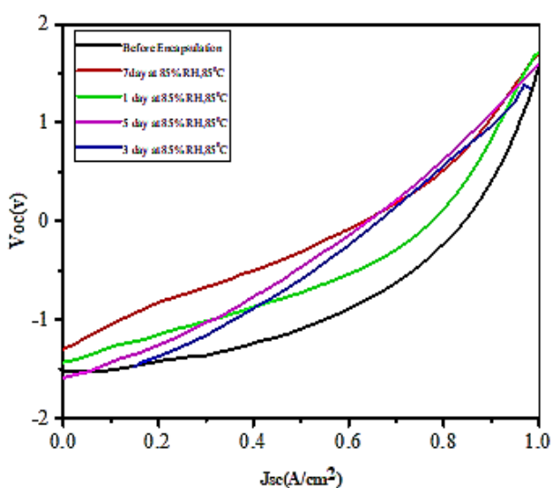
شکل ۲- نمودار جریان ولتاژ سلول خورشیدی کپسول شده با پلی متیل متاکریلات
