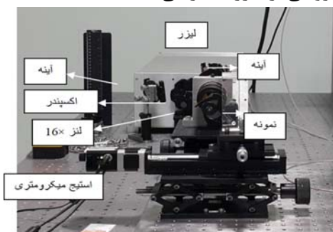
شکل ۱- چیدمان ساخت موجبر لیزری
