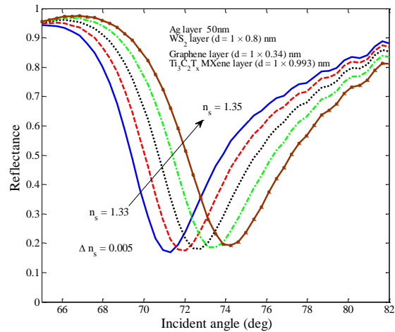
شکل ۳: بازتاب برحسب زاویه نور فرودی با تغییر ضریب شکست محیط حسگری از 1/33 تا 1/35 .
