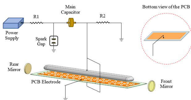
شکل ۲ شماتیک لیزر ساخته شده با سیستم پیش‌یونیزاسیون پلاسمای سطح PCB.
