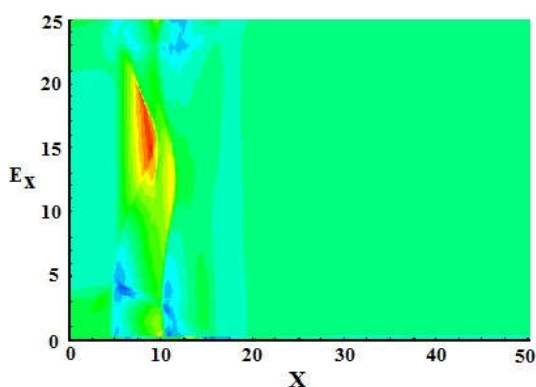
شکل ۳: تحول فضا-زمانی موج پلاسمایی برانگیخته شده در پلازما با \delta=0.2 و B=0.1 در دو زمان \tau=30 و \tau=75 .
