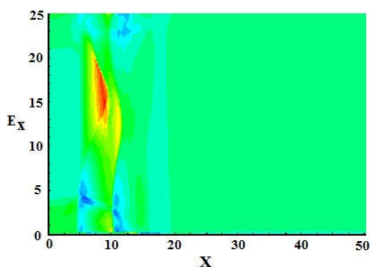
شکل ۳: تحول فضا-زمانی موج پلاسمایی برانگیخته شده در پلاسما با \delta=0.2 و B=0.1 در دو زمان \tau=30 و \tau=75 .
