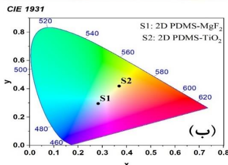
شکل ۳. (الف) توزیع مکانی شدت در نمونه دوبعدی \text{PDMS-MgF}_2 با قرار دادن پخش‌کننده در مسیر اپتیکی و (ب) رنگ‌سنجی از نمونه‌های دوبعدی \text{TiO}_2 و \text{MgF}_2 .
