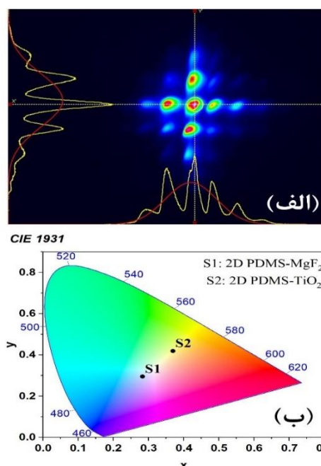
شکل ۳. (الف) توزیع مکانی شدت در نمونه دوبعدی PDMS-MgF 2 با قرار دادن پخش‌کننده در مسیر اپتیکی و (ب) رنگ‌سنجی از نمونه‌های دوبعدی TiO 2 و MgF 2 .
