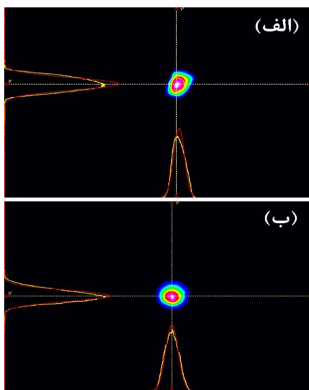
شکل ۲: تصویرهای ثبت‌شده از پروفایل توزیع فضایی شدت نور برای حالت‌های: (الف) قبل و (ب) بعد از قرار دادن پخش‌کننده نوری در مسیر اپتیکی. منحنی‌های زرد رنگ، توزیع شدت اندازه‌گیری‌شده و منحنی‌های قرمز رنگ توزیع شدت گاوسین متناظر در جهت‌های x و y را نشان می‌دهند.
