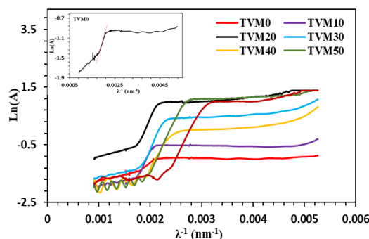
شکل (۶): نمودار \ln(A/\lambda) برحسب (1/\lambda) برای شیشه‌های TVMx. تصویر درونی با خط چین ناحیه‌ی خطی نمودار اورباخ نمونه TVM0 را نشان می‌دهد.
