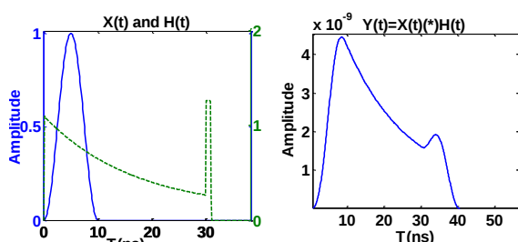
شکل ۳: پاسخ محیط مه و مانع صلب مخفی شده در فاصله ۹m
