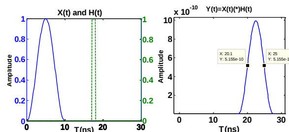
شکل ۱: چپ: شکل پالس و پاسخ محیط، راست: حاصلضرب کانولوشن
