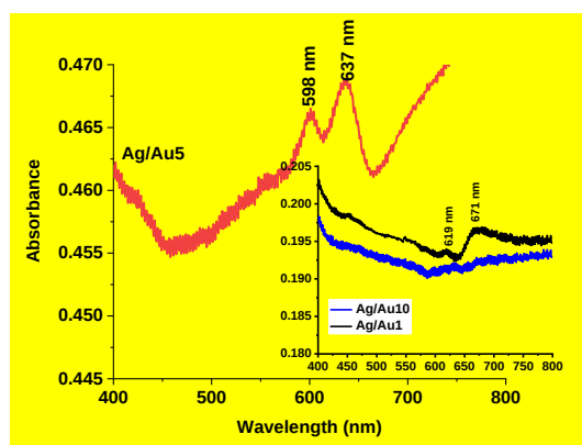
شکل ۲: طیف جذب نمونه‌های Ag/Au5، Ag/Au1 و Ag/Au10. طیف جذب نمونه‌های Ag/Au1 و Ag/Au10 در داخل شکل ۲ نشان داده شده است.
