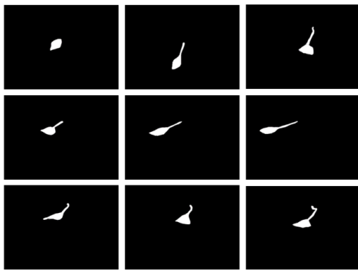
شکل ۶: تصاویر سیاه و سفید برای بررسی میزان کشیدگی.
