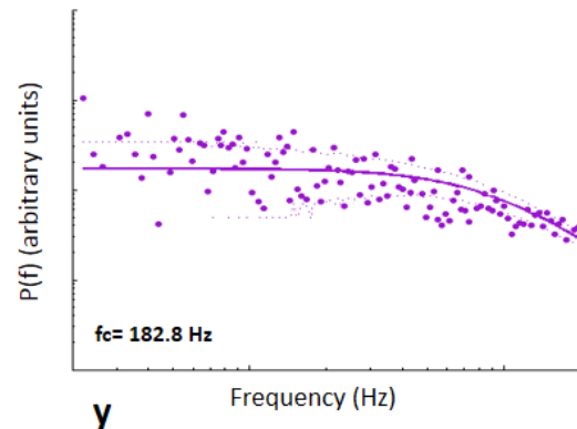
شکل ۴: برازش نمودارهای لورنتسی بر طیف توانی در راستای x و y.
