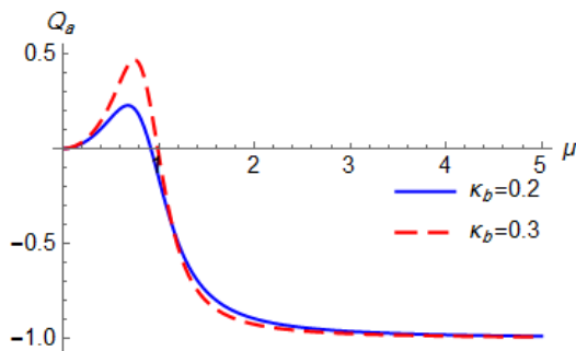
شکل ۱: پارامتر مندل مد a بر حسب \mu برای N=10 ، \kappa_b=0.3 (خط چین قرمز) و \kappa_b=0.2 (خط توپر آبی)
