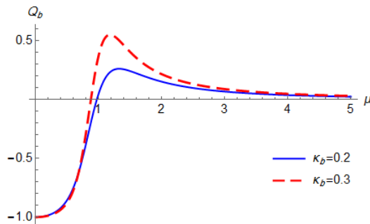
شکل ۲: پارامتر مندل مد b بر حسب \mu برای N=10 ، \kappa_b=0.3 (خط چین قرمز) و \kappa_b=0.2 (خط توپر آبی)
