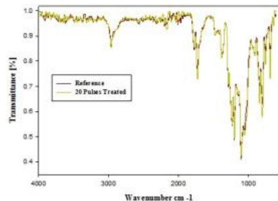
شکل ۳. طیف نشری FTIR لنز قبل و پس از پرتو دهی با لیزر اگزایمر
