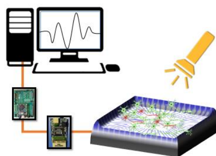
شکل ۱: نمایی از ترکیب روش اپتوژنتیک با ثبت الکتروفیزیولوژی توسط آرایه اپترودی
