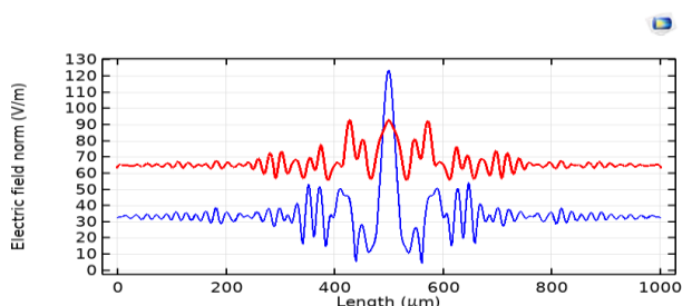
شکل 3: نمودار cut line برای طول موج 20 \mu\text{m} - نمودار قرمز رنگ عدم حضور سلول های توموری و نمودار آبی رنگ برای حالت توموری کردن سلول ها می باشد.
