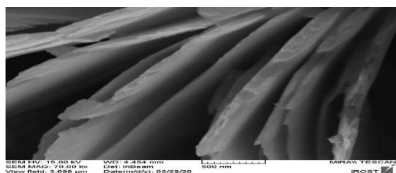
شکل ۴: تصویر میکروسکوپ الکترونی روبشی گسیل میدانی نمونه سنتز شده در ۲۴ ساعت
