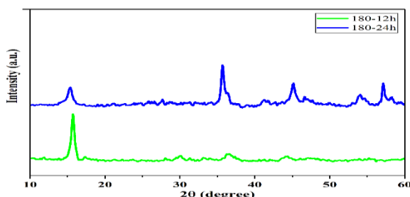
شکل ۱: الگوی پراش اشعه ایکس نمونه ها
