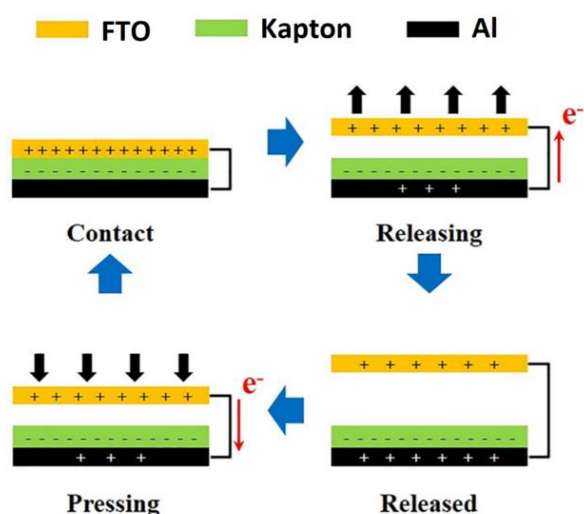
شکل ۲: نحوه تولید جریان به کمک نانومولد تریپوالکتریک در اثر اعمال ضربه.
