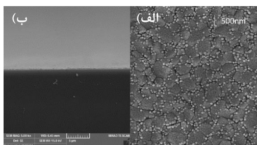
شکل ۲: تصویر FESEM (الف) نمای بالا (top)، (ب) سطح مقطع (cross-sectional) لایه پروسکایت در دمای ۸۰ درجه سانتیگراد.
