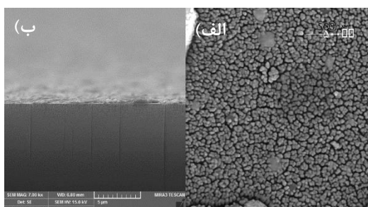
شکل ۴: تصویر FESEM (الف) نمای بالا، (ب) سطح مقطع لایه پروسکایت در دمای ۱۵۰ سانتیگراد.
