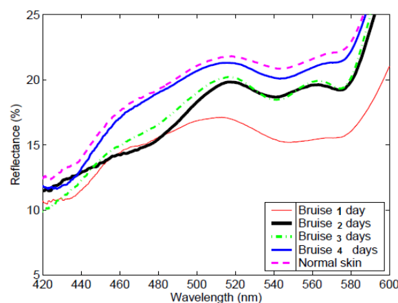
شکل ۶- همان شکل ۵ با زوم بیشتر برای مشخص تر شدن طیف‌ها
