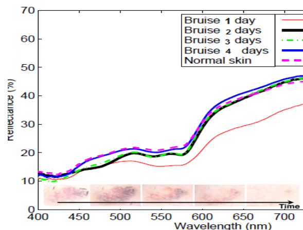
شکل ۵- طیف بازتابی کبودی در ناحیه بازو در گذر زمان
