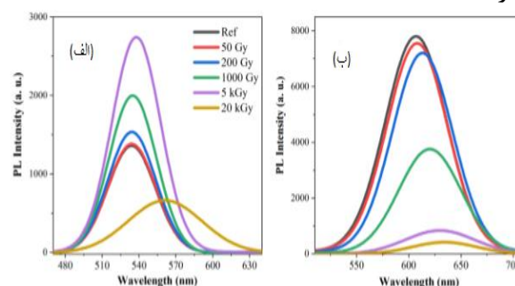
شکل ۴. الف) طیف نوری قبل و بعد از قرار گرفتن در معرض گاما برای (ب) \text{CdTe/CdSe/CdS} و \text{CdTe}
