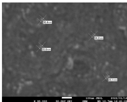
شکل ۳: تصویر میکروسکوپ الکترونی بازتابی از نمونه کیتوسان/نانوپلی آنیلین-طلا.
