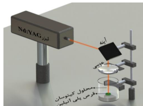
شکل ۱: چیدمان کند و سوز لیزری برای سنتز نانو ذرات پلی آنیلین و طلا در محلول رقیق شده کیتوسان.
